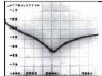
典型80-120YF 型之濾波功能, dB-頻率曲線
