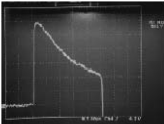
典型箝位電壓波形: 施加3KA 衝擊電流(8/20uS)於80-120Y
